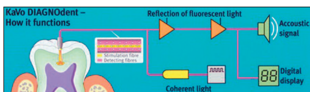
Obr. 2. Schéma funkce laserového fluorescenčního přístroje DIAGNOdent.
