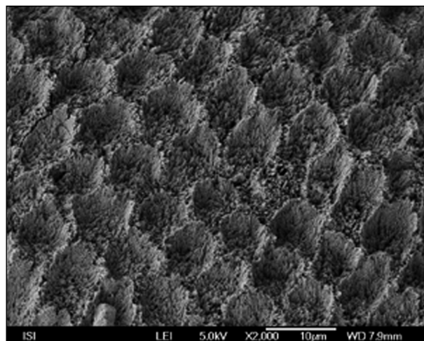
Obr. 2. Vzhled skloviny po předchozím zábrusu skloviny po leptání gelem 37% kyseliny ortofosforečné. Povrch je pravidelný, jde o intraprizmatický způsob naleptání.
