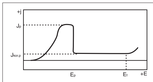
Graf 6. Polarizační křivka kovu přecházejícího do pasivního stavu: E_p – pasivační potenciál, E_t – transpasivační potenciál, j_p – kritická pasivační proudová hustota, j_{kor.p} – korozní proudová hustota v pasivním stavu.
