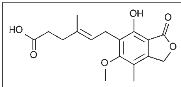
Obr. 3. Strukturní vzorec kyseliny mykofenolové.
