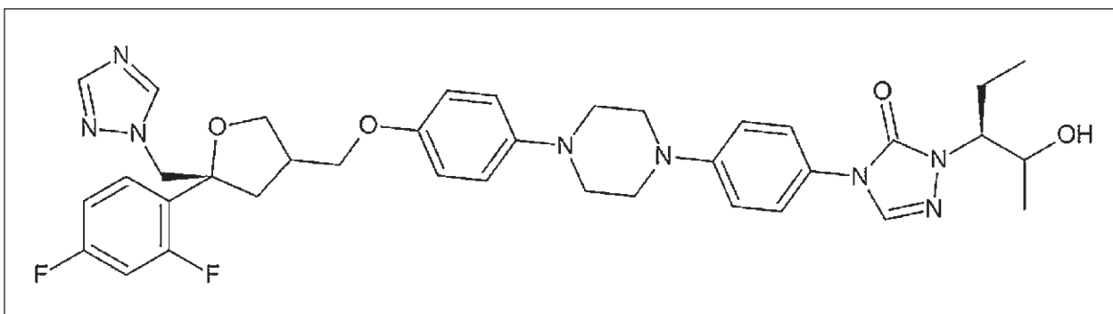
Obr. 5. Strukturní vzorec posakonazolu.
