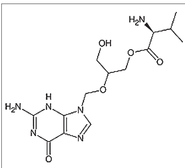
Obr. 6. Strukturní vzorec valgancikloviru.
