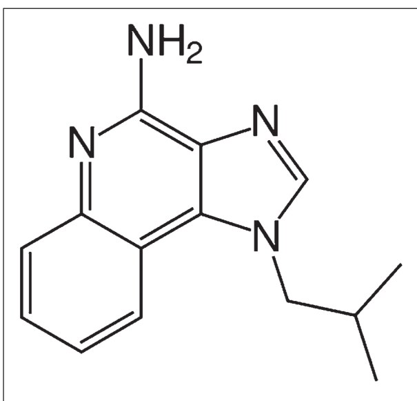
Obr. 1. Strukturní vzorec imiquimodu.
