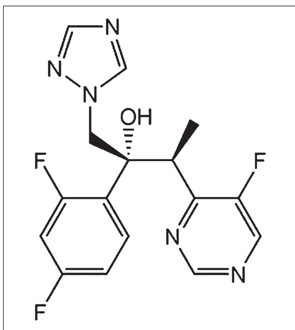
Obr. 4. Strukturní vzorec vorikonazolu.
