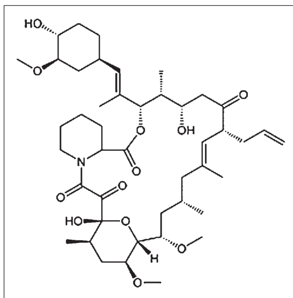
Obr. 2. Strukturní vzorec takrolimu.
