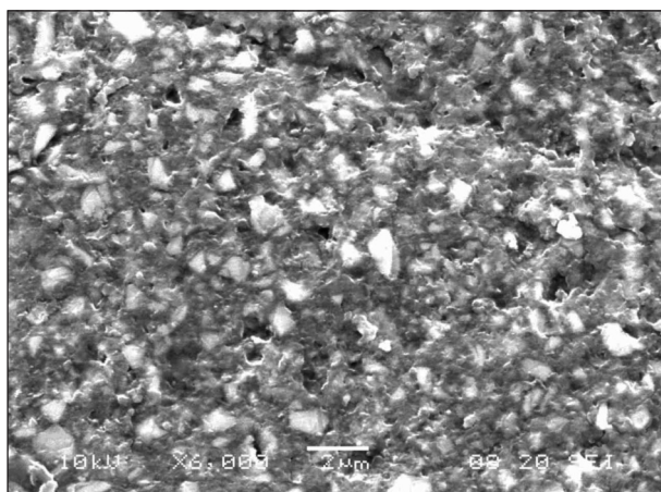
Obr. 3. Povrch kompozitního materiálu a) 2 měsících expozice v destilované vodě, b) po 25 aplikacích bělicího gelu.
